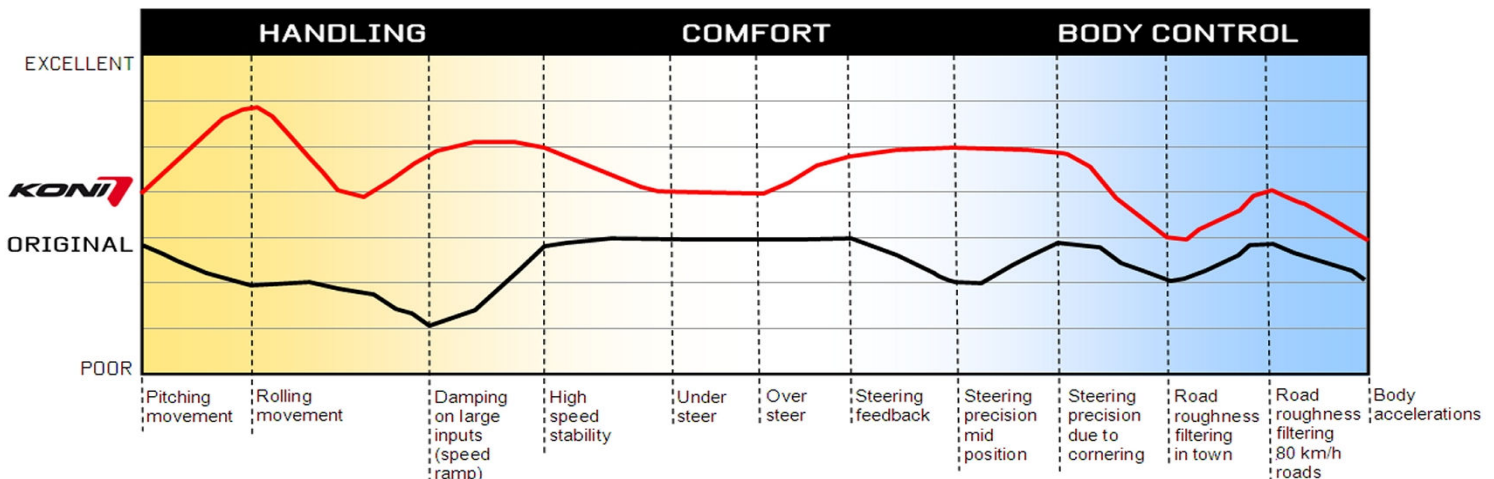
VOLVO C30 - Confronto fra ammortizzatori originali e KONI FSD (fonte: KONI Ride & Handling Center)
